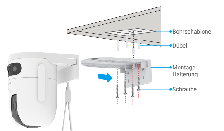
Abb. 1 Deckenmontage
